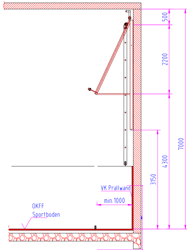
Gitterleiter
